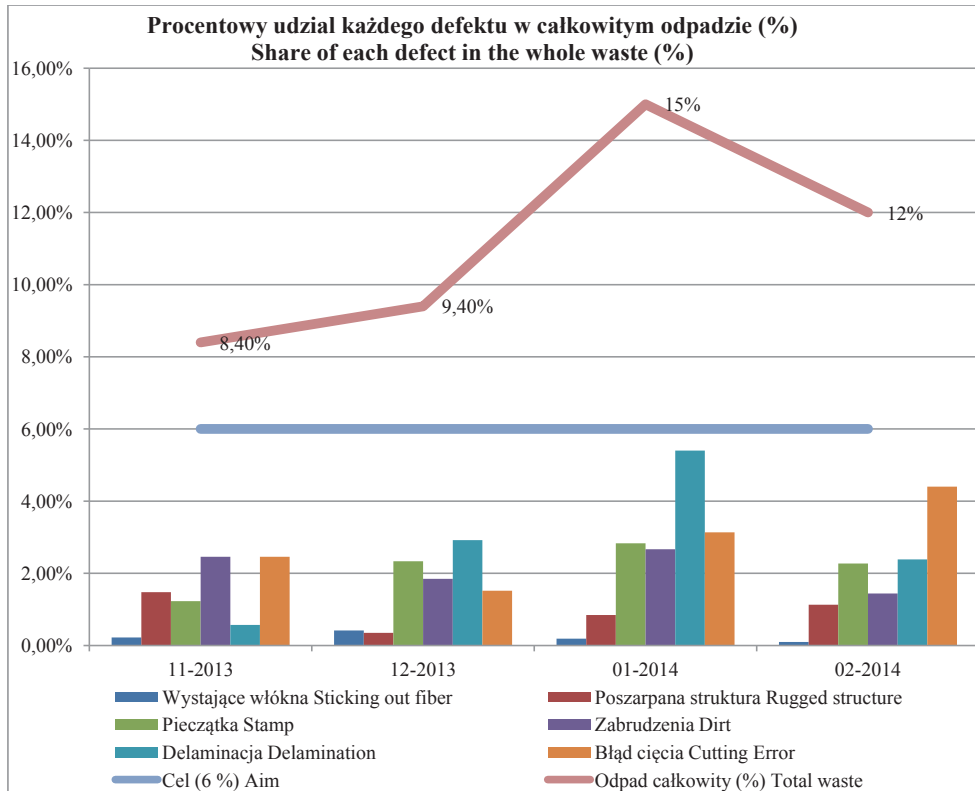
Rys. 1. Procentowy udział każdego defektu w całkowitym odpadzie Fig. 1. Share of each defect in the whole waste (%)
