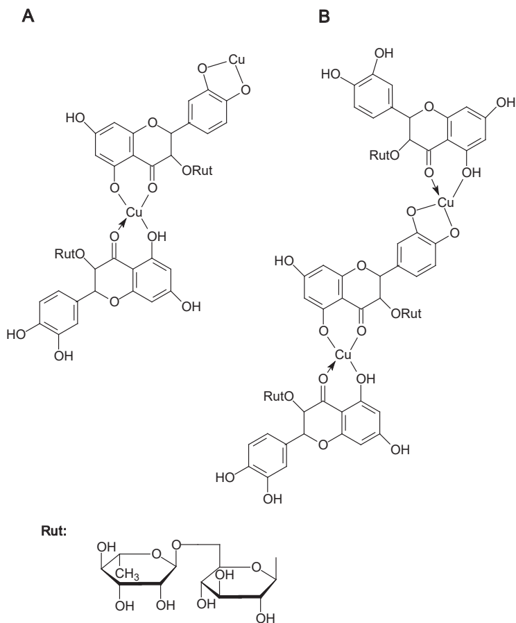
Rysunek 13. Przepuszczalne struktury kompleksów rutozydu z jonami miedzi(II) [25]
