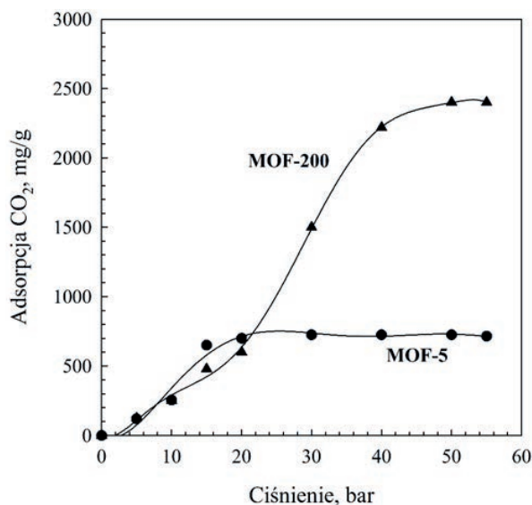
Rysunek 5. Izotermy adsorpcji \text{CO}_2 zmierzone na MOF-5 i MOF-200 w temperaturze 25^\circ\text{C} . Na podstawie zezwolenia, wykonano rysunek z pracy [42]. Prawa autorskie ® 2010 należą do American Association for the Advancement of Science
