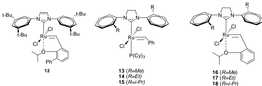
Rysunek 19. Struktury katalizatorów, które okazały się użyteczne w metatezie tetrasubstytucjonowanych olefin Figure 19. Structures of catalysts that have proved to be useful in tetrasubstituted olefin metathesis
