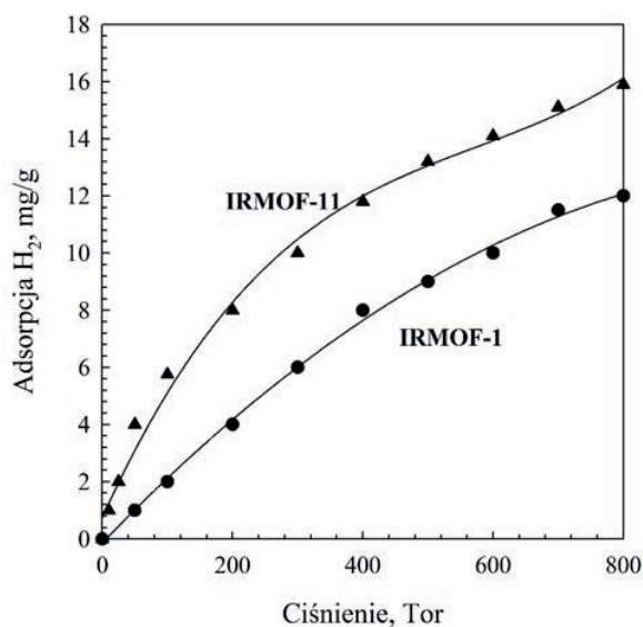
Rysunek 7. Izotermy adsorpcji H_2 w temperaturze -196^\circ\text{C} na IRMOF-1 i IRMOF-11. Na podstawie zezwolenia, wykorzystano rysunek z pracy [64]. Prawa autorskie ® 2004 należą do American Chemical Society
