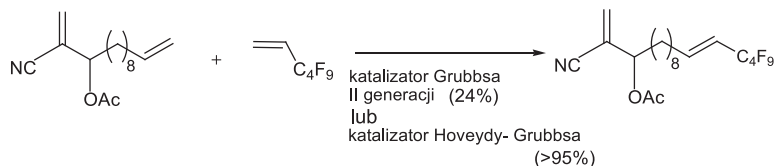
Rysunek 10. Schemat reakcji metatezy, w której substratem jest fluorowana olefina, katalizowanej katalizatorem Grubbsa II generacji lub katalizatorem Hoveydy- Grubbsa.
