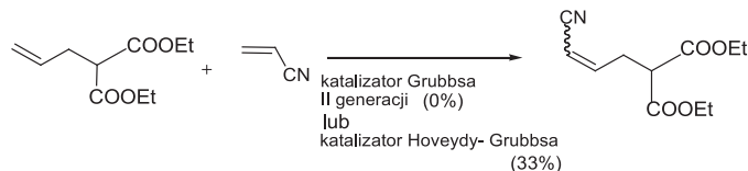
Rysunek 9. Schematy reakcji metatezy akrylonitrylu katalizowanej katalizatorem Grubbsa II generacji z wydajnością 0% lub katalizatorem Hoveydy-Grubbsa z wydajnością 33%
