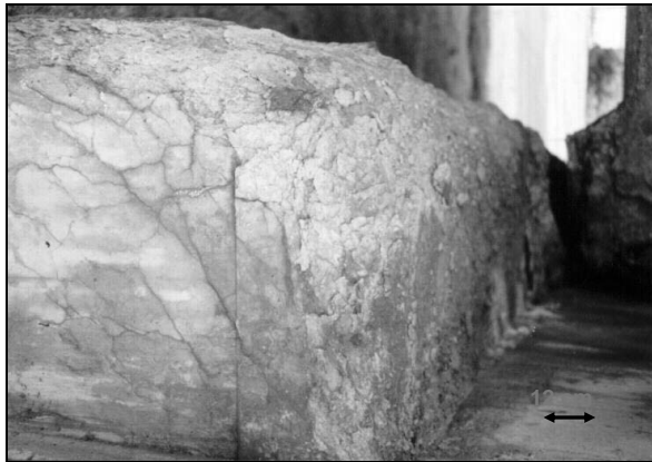
Rys. 6. Wiadukt k. Kielce. Destrukcja elementów betonowych wywołana reaktywnością alkaliczną. Odpryskiwanie i łuszczenie się betonu. Widoczne wycieki żelowe oraz rdzawe nacieki pochodzące od korodującego odkrytego zbrojenia (Góralczyk, 2000)
