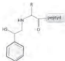
Schemat 18. Grupa 2-merkapto-2-fenyletylowa
