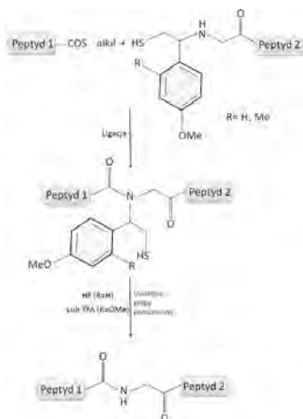
Schemat 16. Reakcja ligacji z zastosowaniem grupy N^{\alpha} -1-arylo-2-merkaptoetylowej Scheme 16. Ligation reaction using N^{\alpha} -1-aryl-2-mercaptoethyl group
