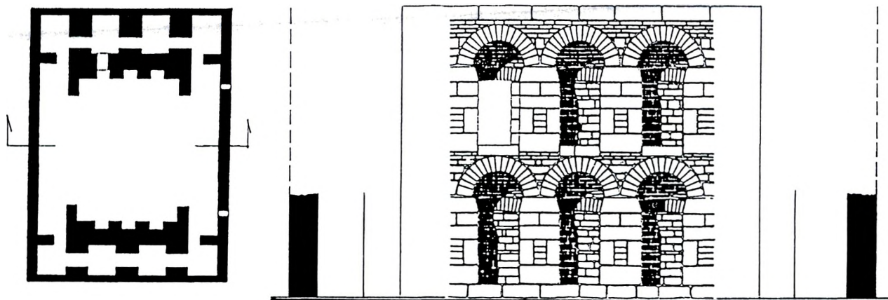
Ryc. 19. Nysa – biblioteka, rzut i przekrój (wg [1, s. 235])
