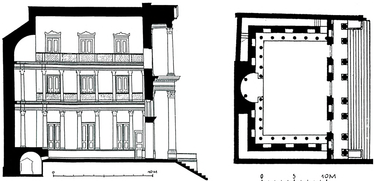
Ryc. 14. Efez – biblioteka, rzut i rekonstrukcja przekroju (wg [30, il. 109]; [19, s. 56])
