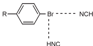
Schemat 3. Schemat badanych układów z pochodnymi bromobenzenu
