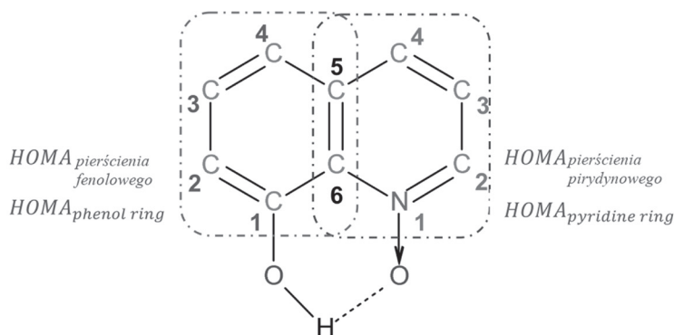
Rysunek 5. Struktura molekularna N -tlenku 8-hydroksychinoliny z nomenklaturą pierścieni aromatycznych użytą w analizie HOMA
