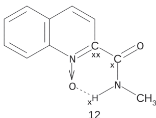
Rysunek 6. Struktura molekularna pochodnej N-tlenku chinoliny dla której wykonano obliczenia NMR. x – oznacza atomy dla których policzono przesunięcia chemiczne
