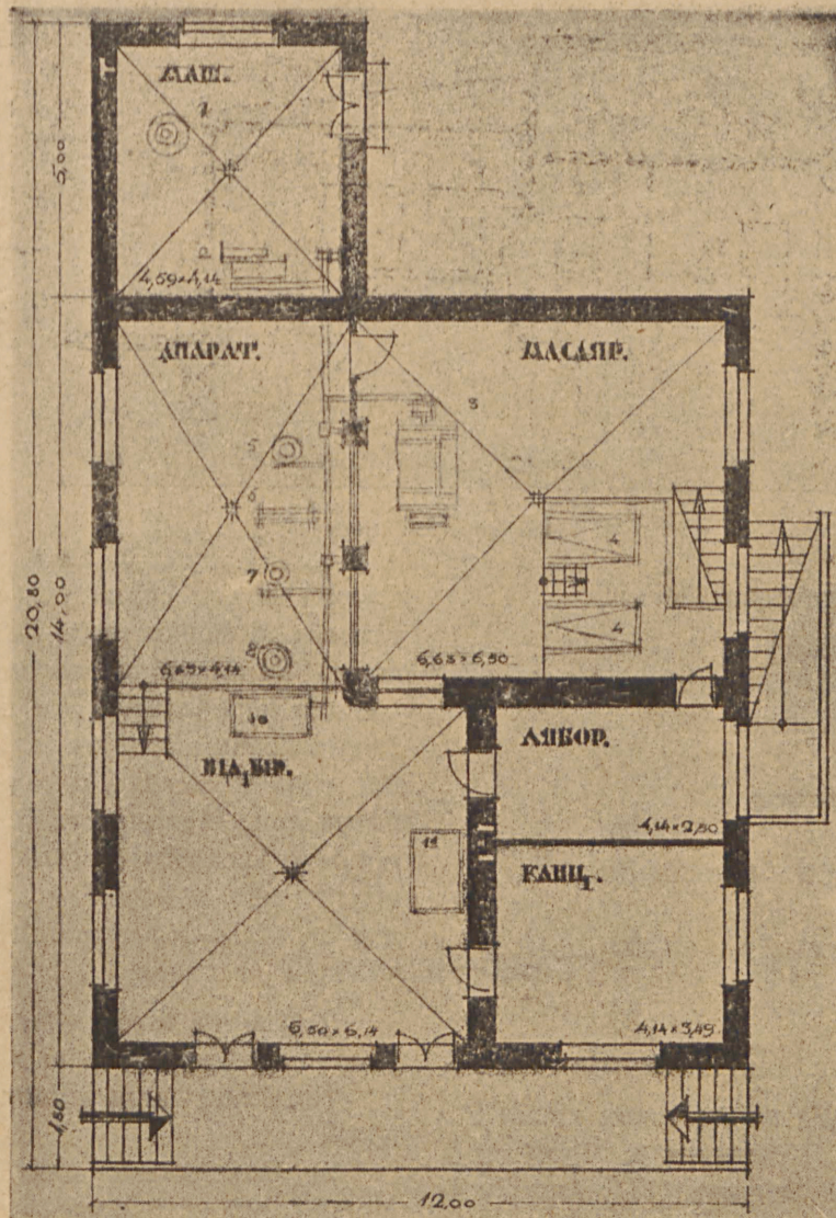
Плян партеру.
